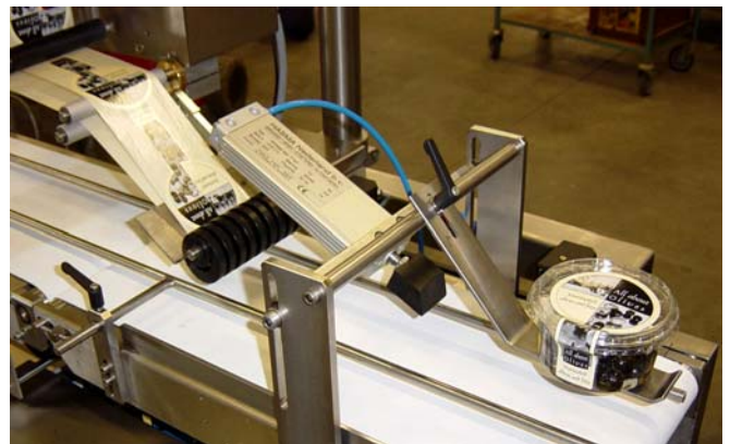
Een etikettendispenser voor het aanbrengen van diverse etiketvormen en etiketten met sluitzegel.
