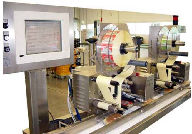
Sandwich verpakkingen en belegde broodjes op boven- en onderzijde etiketteren. Productielijn incl. 100% barcodecontrole en metaaldetector.
